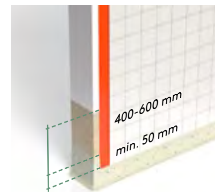
FIGUR 10. Mekanisk förankring av tätskikt (typ 2).
