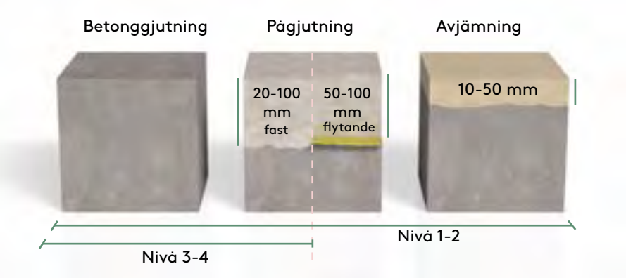
FIGUR 1. Massiva underlag
