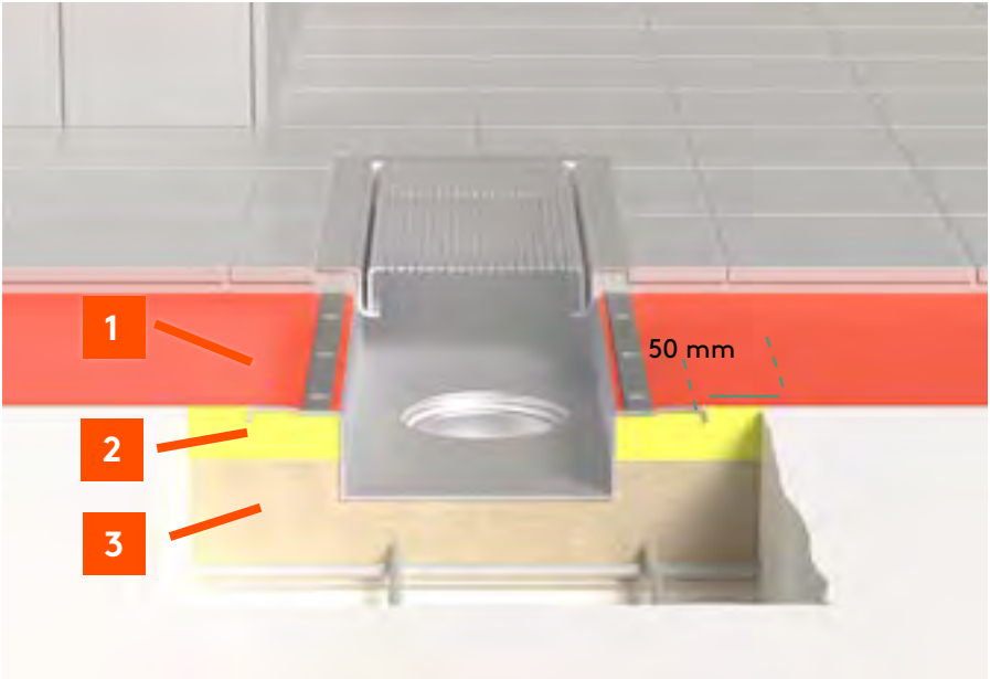
FIGUR 12. Typlösning för brunn i Storkök (1) Tätskikt, (2) Kapillärbrytare, (3) Gjutning i ursparning.
