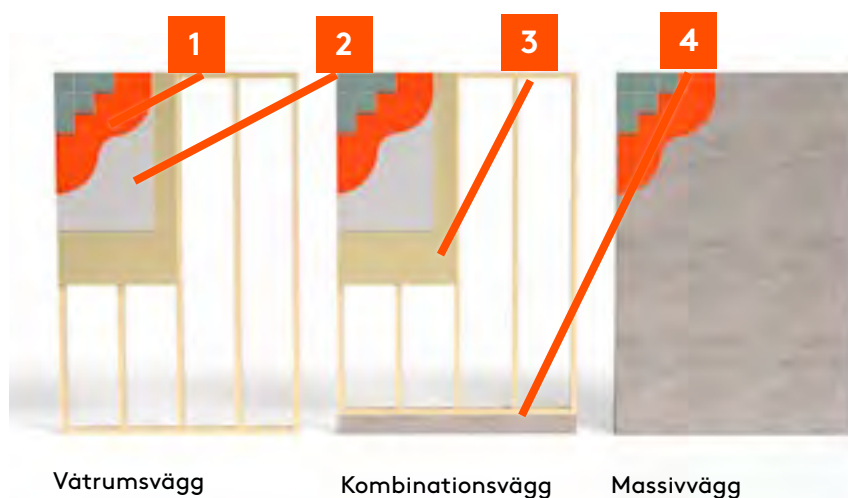
FIGUR 13. Väggtyper. (1) Tätskikt, (2) Skiva, (3) 15 mm plywood, (4) Sockel
