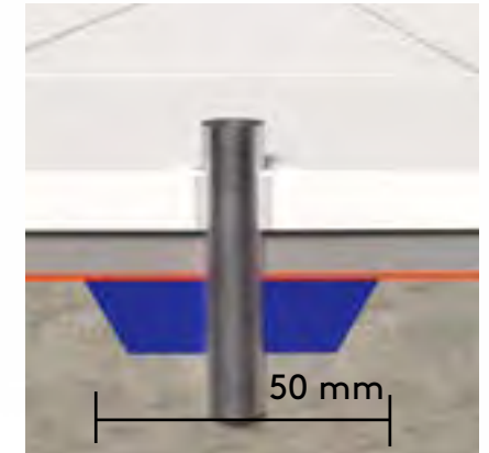
FIGUR 5. Kapillärbrytare
