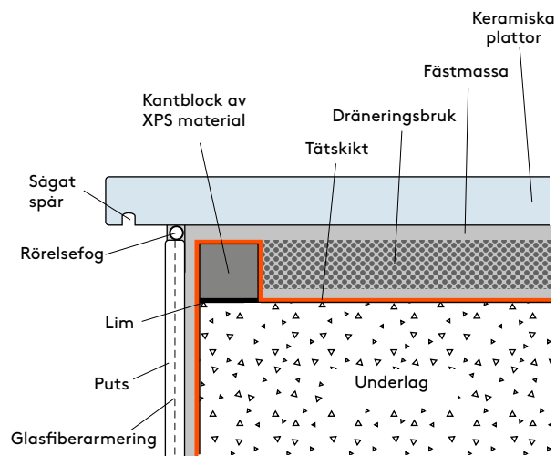
BILD 12. Trappa – Plansteg
