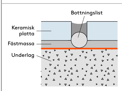
BILD 9. Bottningslist och bottningsstejp är hjälpmedel för att undvika kontakt mellan fogmassa och underlaget samt ge rörelsefogen rätt utformning.
