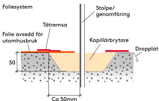
BILD 6. Foliesystem avsett för utomhusbruk
