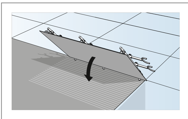
BILD 15. Exempel på montering av golvplattor.
