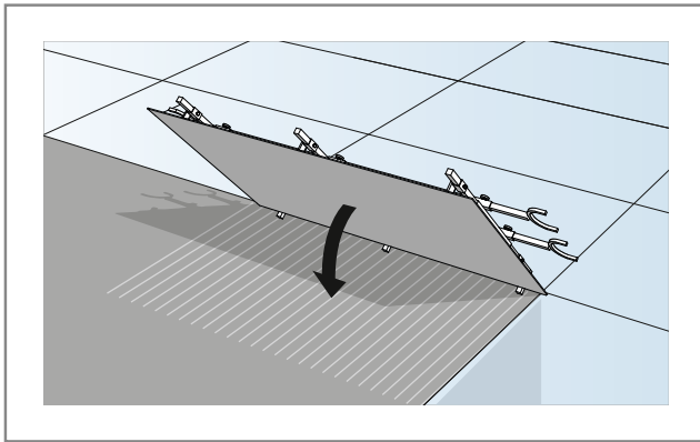
BILD 14. Exempel på montering av golvplattor.
