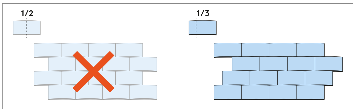
BILD 3. Vid rektangulära plattor kan fogsprången överstiga gränsen satt i Byggherakamirådets Riktlinjer för färdigt utförande om 1/3 förband tillämpas.
