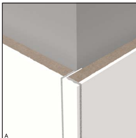
FIGUR 18 A. Kantlist
