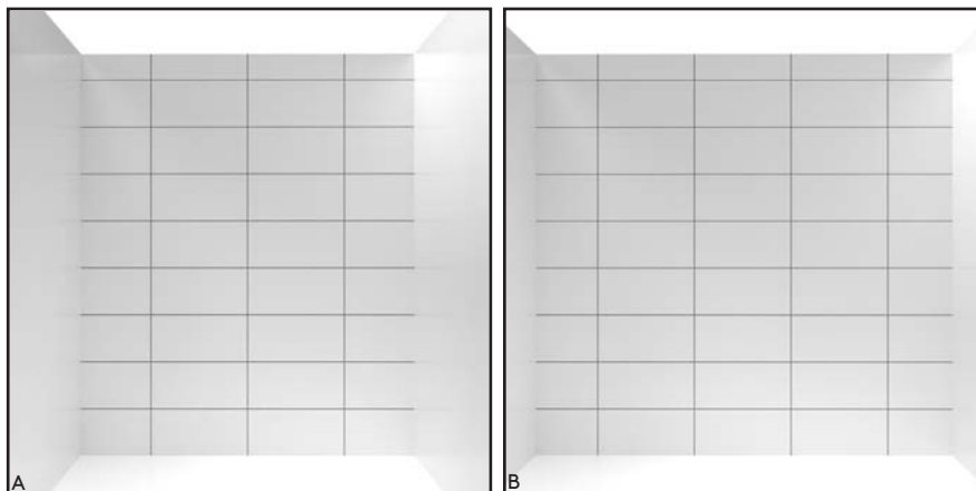
FIGUR 3 A-B. Där väggen styr centreringen gäller att passbitarna in mot hörnen bör vara minst \frac{1}{3} av plattan. Detta hanteras genom att låta fogen centrera eller låta plattan centrera.
